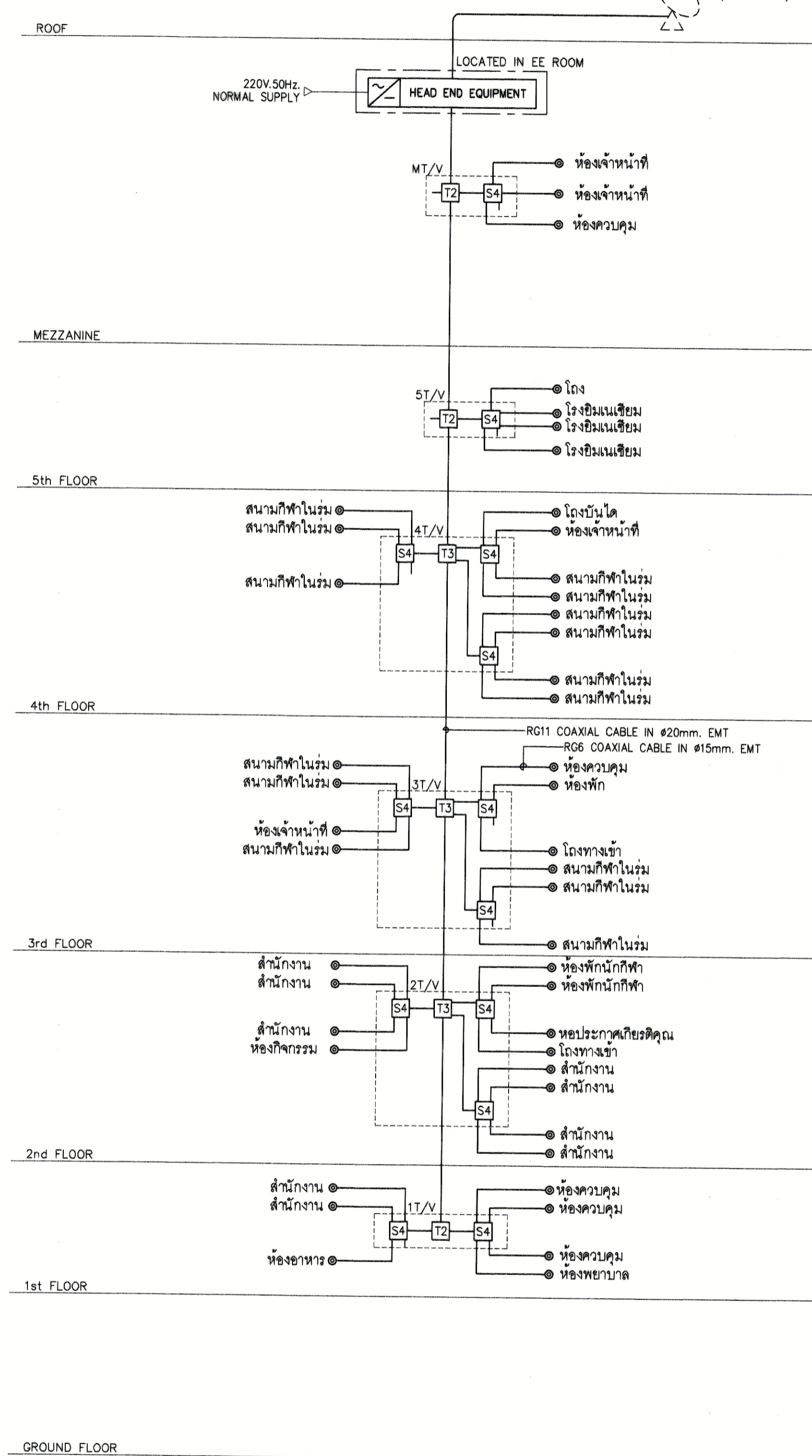
ไอเซอริไดอะแกรมระบบโทรทัศน์รวม
