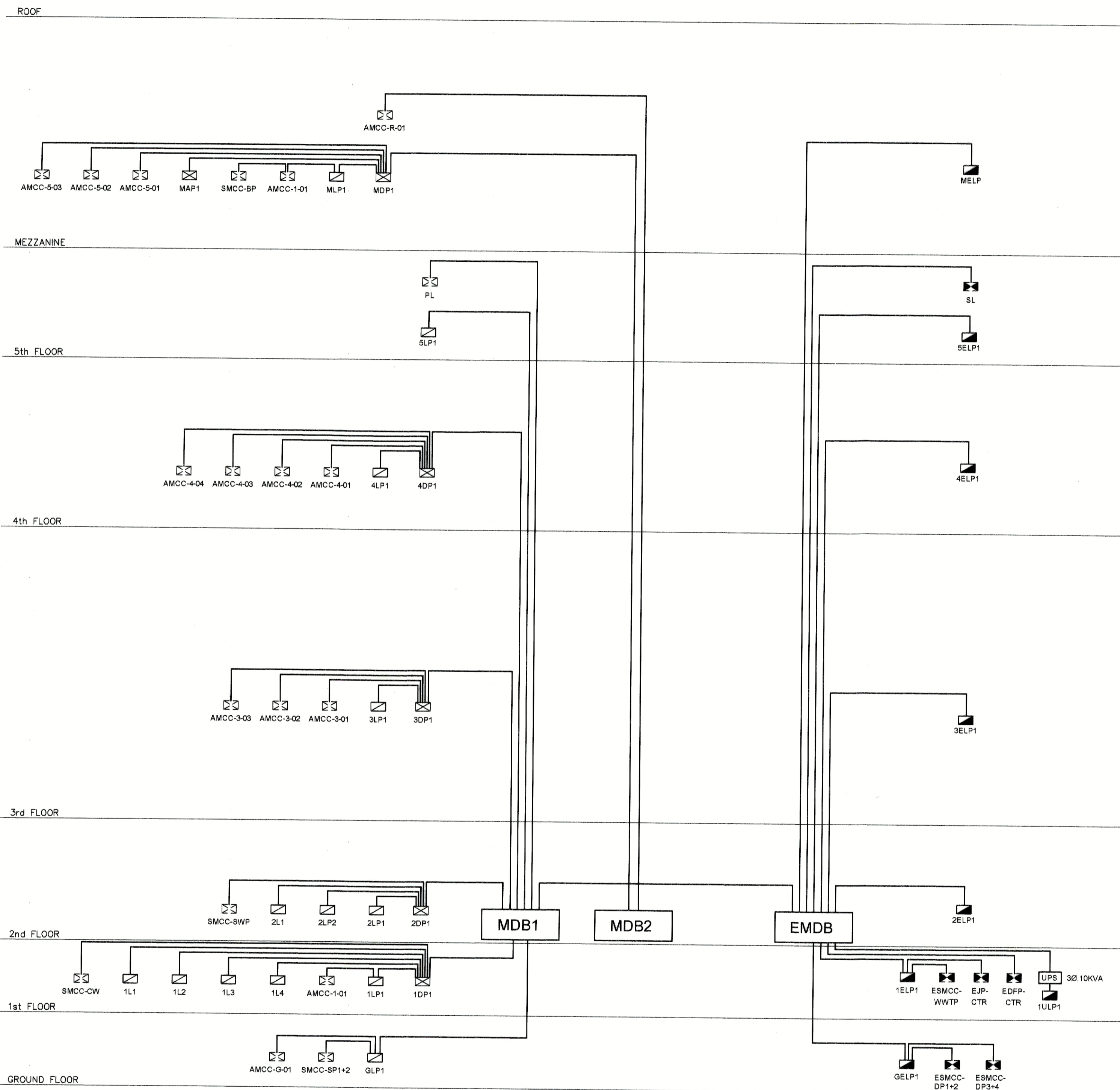
ไอเซอริไดอะแกรมระบบไฟฟ้า
