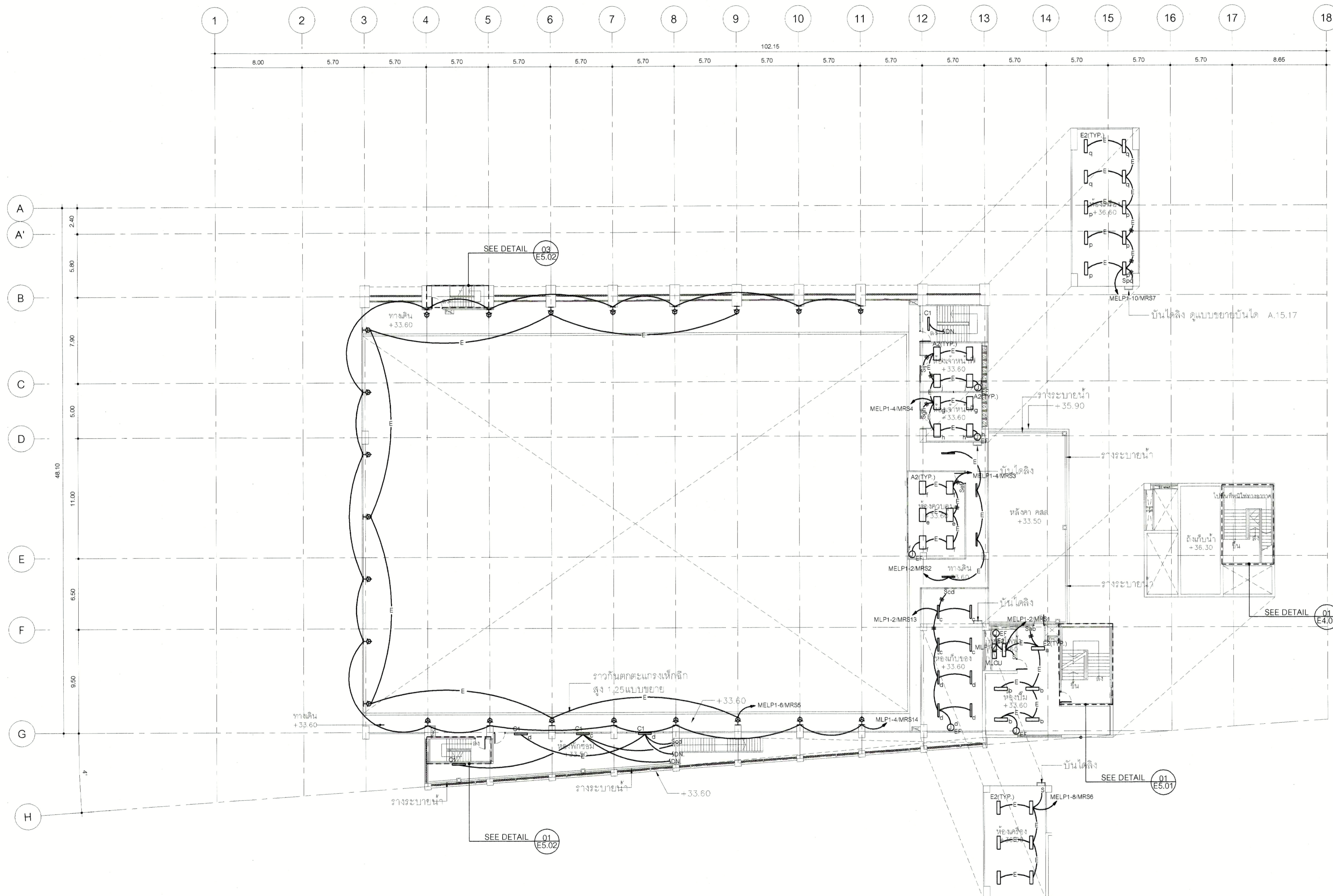
ผังระบบไฟฟ้าแสงสว่าง ชั้นลอย SCALE 1 : 200
